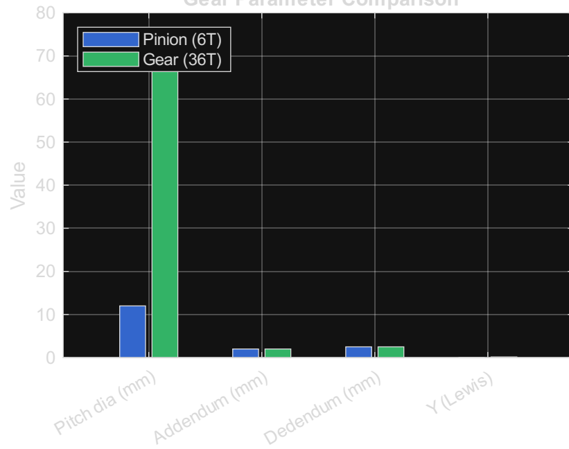
Gear Parameter Comparison
